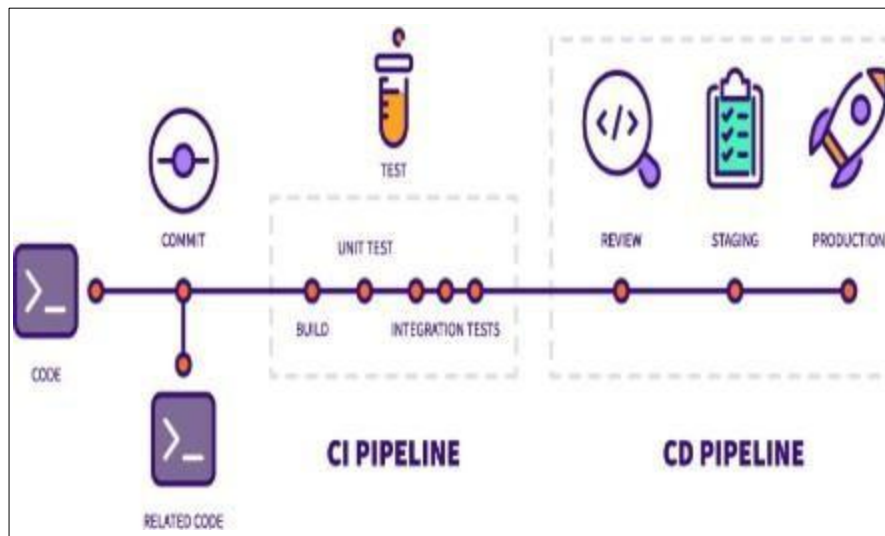
Figure 5 Modernizing CI/CD using GITLAB CI
